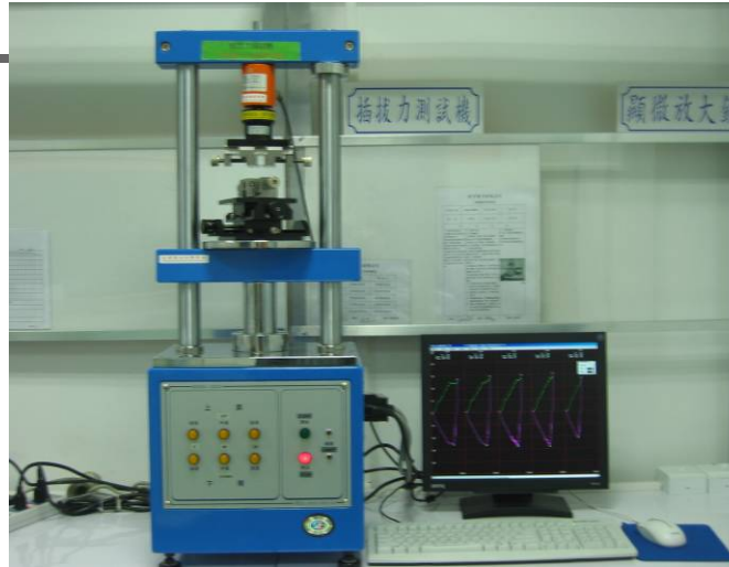
插拔力測試機 Mating/un-mating Tester
